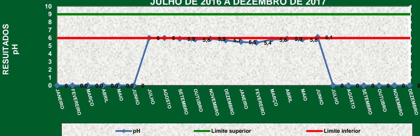
pH NASCENTE GADO 2 JULHO DE 2016 A DEZEMBRO DE 2017
