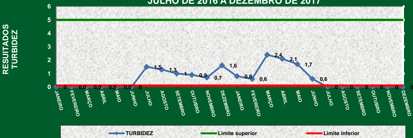
TURBIDEZ NASCENTE GADO 2 JULHO DE 2016 A DEZEMBRO DE 2017
