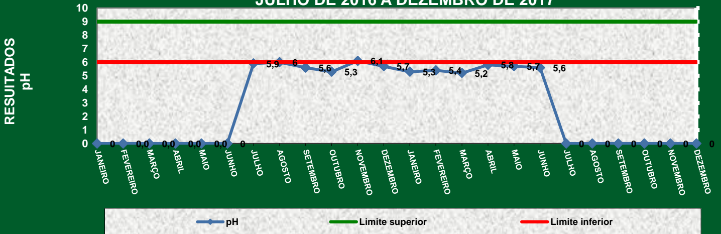
pH NASCENTE REPRESA DO JAMIL JULHO DE 2016 A DEZEMBRO DE 2017
